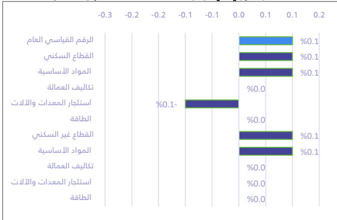
شكل 5: التغير الشهري في مؤشر تكاليف البناء حسب القطاع و الأقسام (%)
