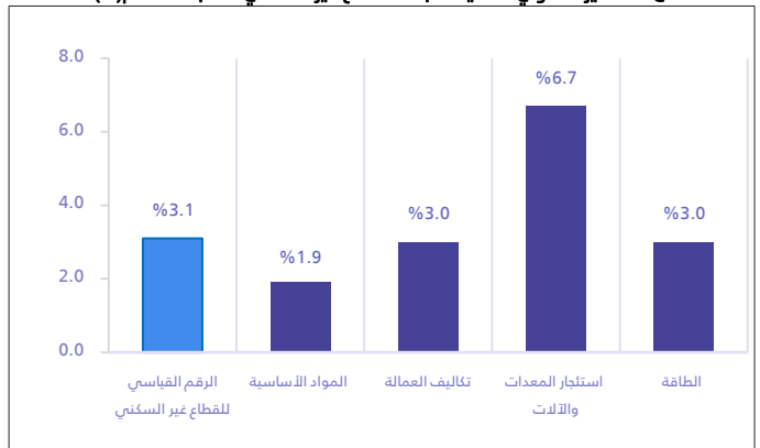
شكل 3: التغير السنوي لتكاليف البناء للقطاع غير السكني حسب الأقسام (%)
